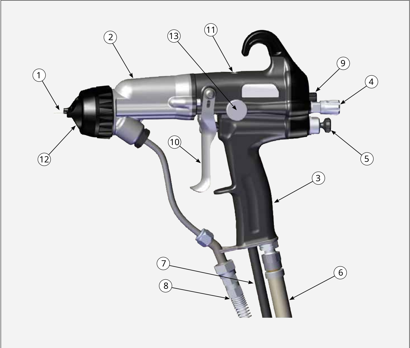
Рисунок 1: Электростатический распылитель на основе растворителя Ransflex 81545 / 81565
