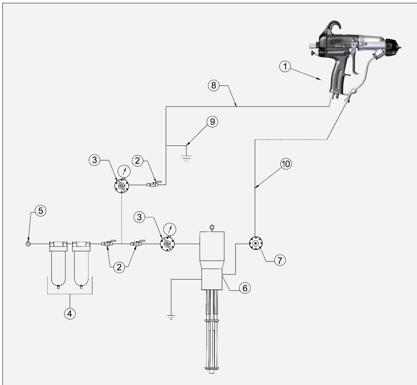
Рисунок 2: Типичная установка Ransflex на основе растворителя
