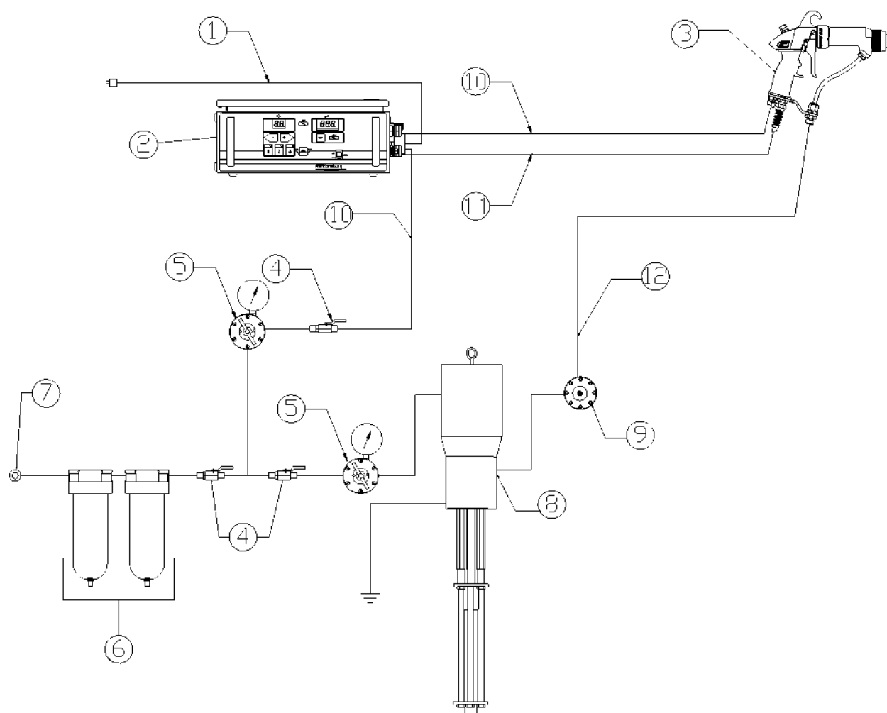
Рисунок 3: Типичная установка аппликатора краски на основе растворителя
