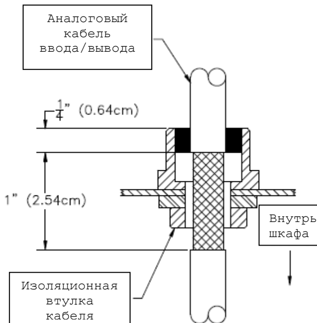
Рис. 6. Изоляционная втулка кабеля
