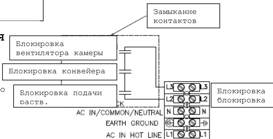
Рис.9а. проводка блокировки
