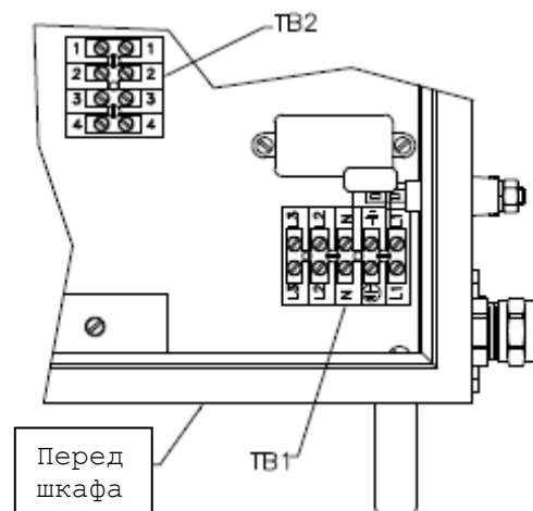
Рис. 8. расположение TB1 и TB2 d источнике питания
