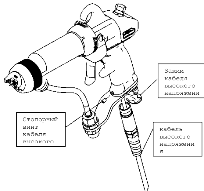
Рисунок 10: Снятие и установка кабеля высокого напряжения
