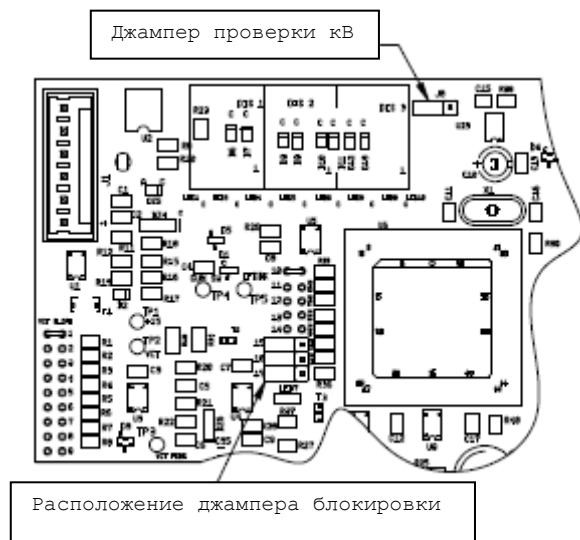
Рисунок 16: расположение джампера блокировки
