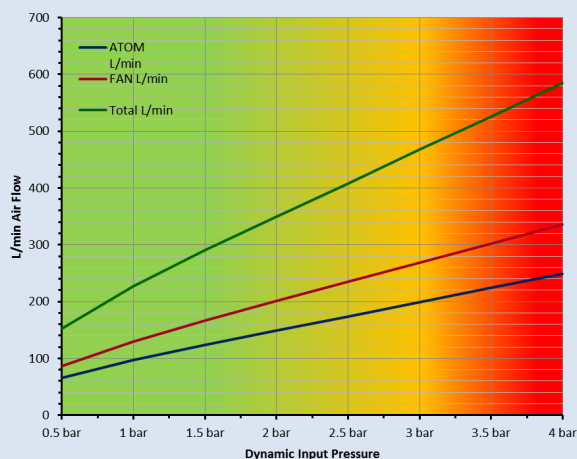
TE40 Air Cap
