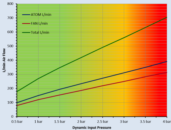
TE50 Air Cap
